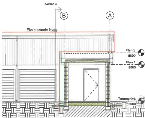
Snitt A 1 : 50
