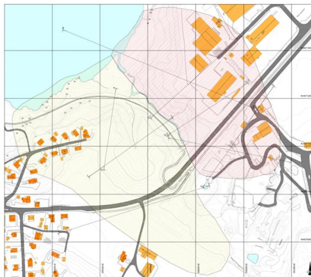
Skredfareområder markert med gult og rødt (Kart fra geoteknisk rapport "Gatedalen Miljøanlegg", Multiconsult, 29.06.2022)
